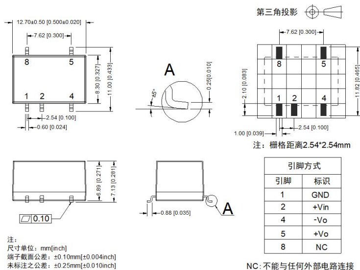
封装尺寸图
